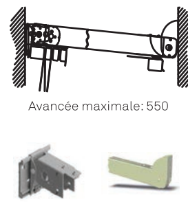
Fixation Face
